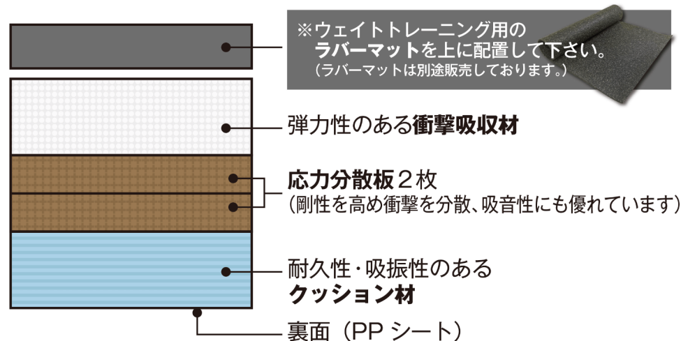
ラバーマット(別売)
